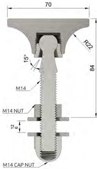
Ø70 UV Yapıştırılmalı Hareketli Rotil Ø70 UV Glass Bonding Swivel Routel
